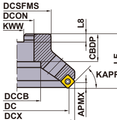
Fig.3 ø125
