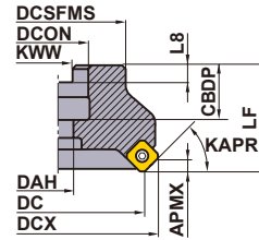
Fig.1 ø50 ø63
